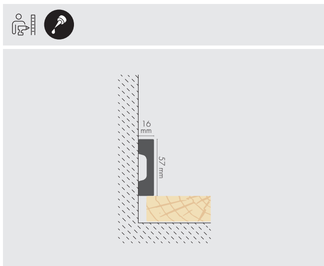
LPC-27 LISTWA PRZYPODŁOGOWA SKIRTING BOARD SOCKELLEISTE
