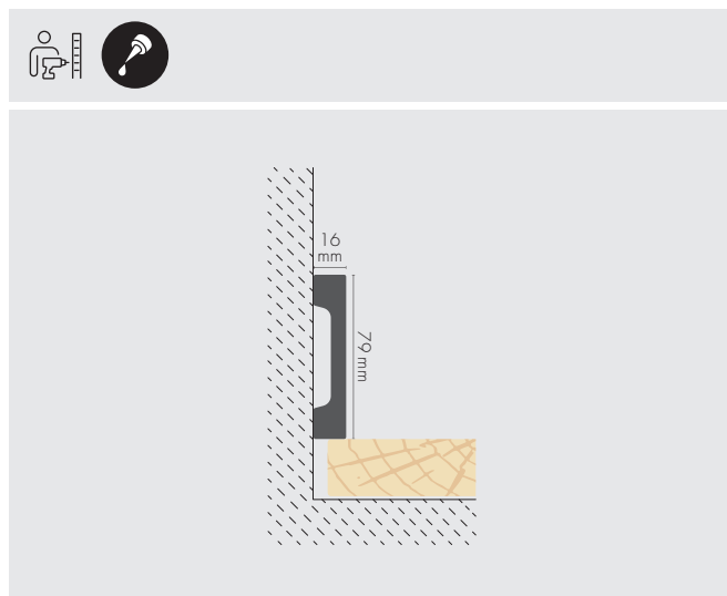
LPC-28 LISTWA PRZYPODŁOGOWA SKIRTING BOARD SOCKELLEISTE
