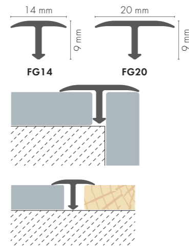
FG14/ FG20 ALU
