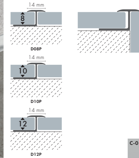
D08P/ D10P/ D12P ALU
