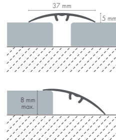
LW47C5W1 ALU
