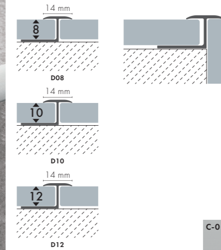
D08/ D10/ D12 ALU
