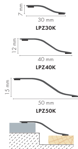
LPZ30K/ LPZ40K/ LPZ50K ALU
