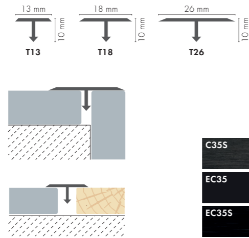
T13/ T18/ T26 ALU
